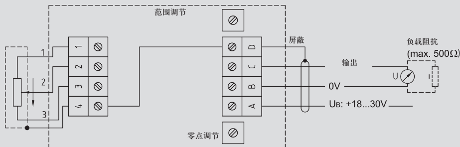
接线图
